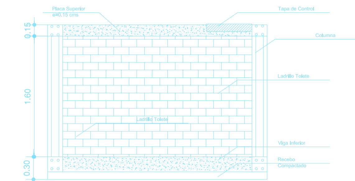
CORTE GRAL. TANQUE
