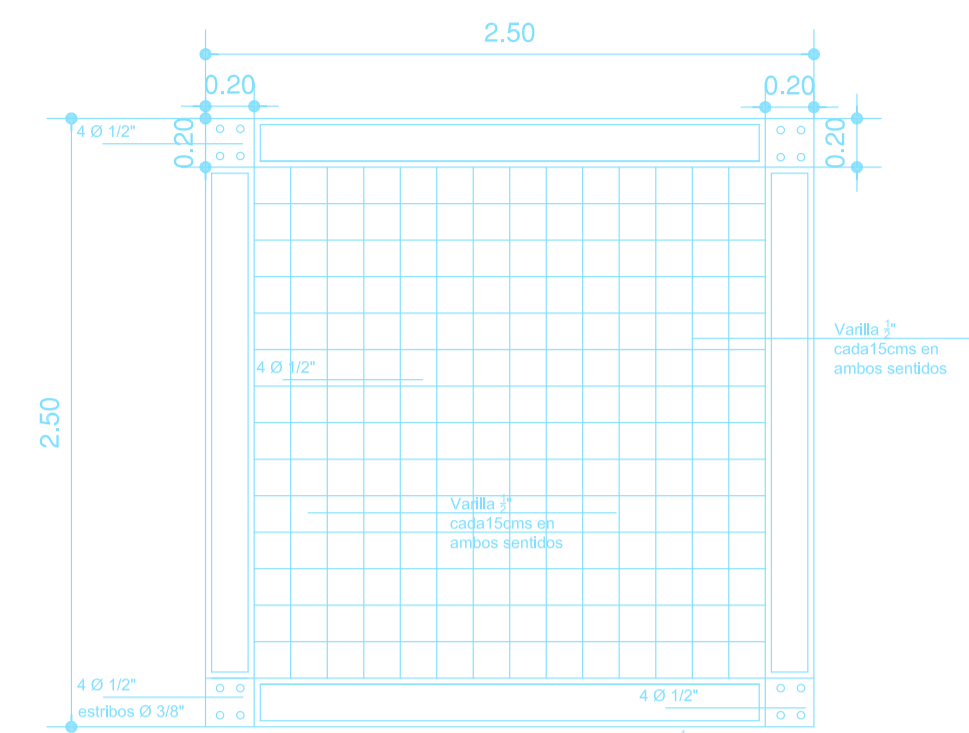
PLACA INFERIOR
