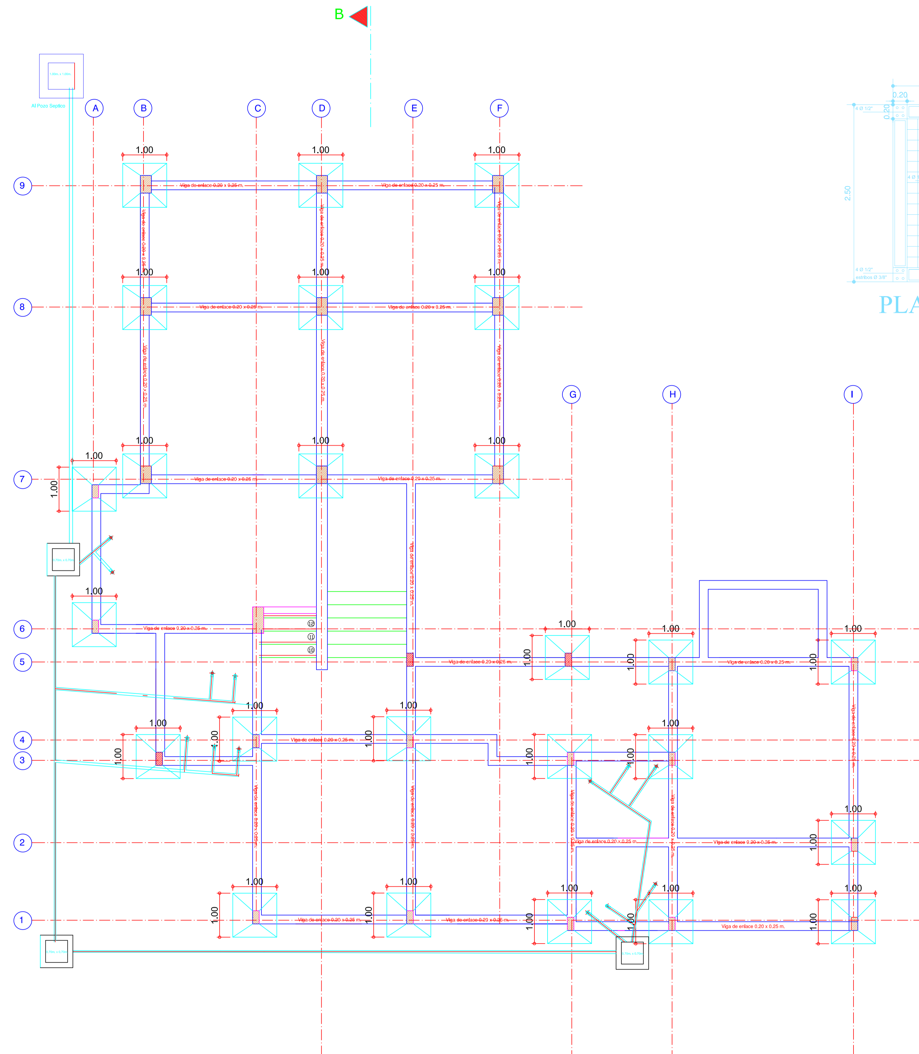
EJES, CIMIENTOS Y DESAGUES
