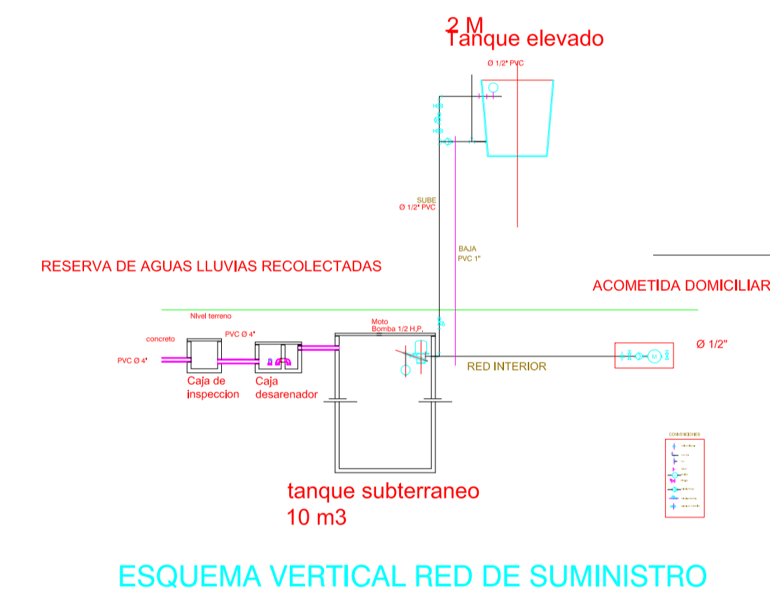
ESQUEMA VERTICAL RED DE SUMINISTRO
