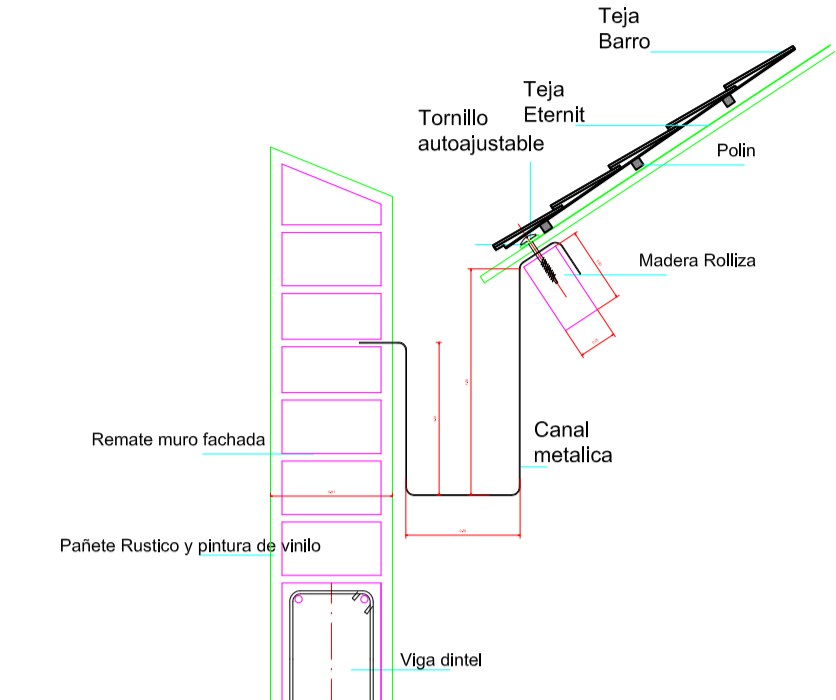
DETALLE REMATE CUBIERTA
