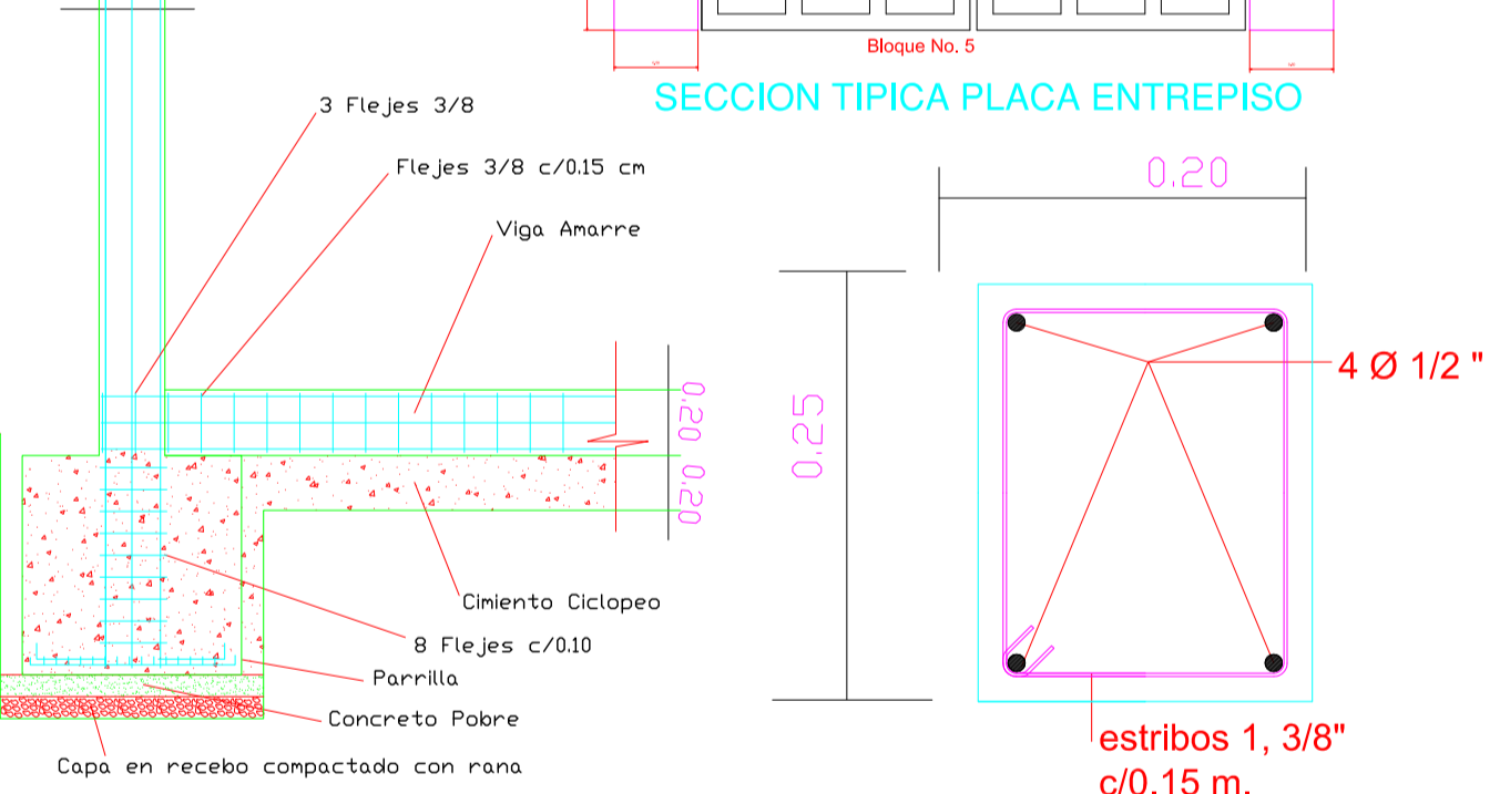
DETALLE FLEJE TIPICO COLUMNAS ESC. 1:10
